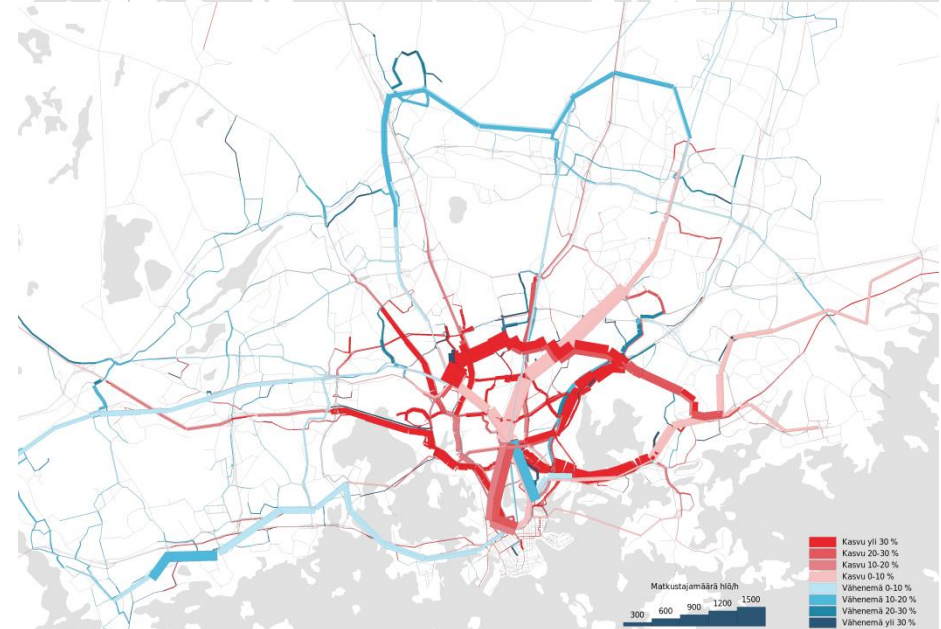
Vaikutukset tieliikenteen ja joukkoliikenteen määriin aamuruuhkassa, ve 3.
