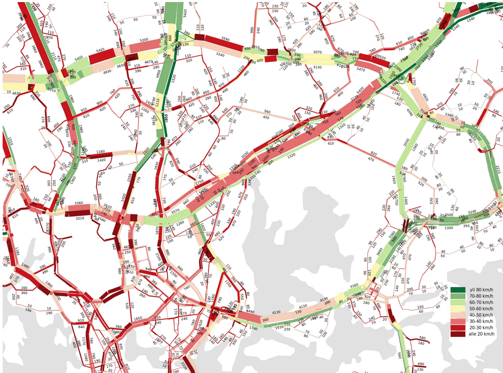
Autoliikenteen määrät ja sujuvus, AHT 2050 ve Lb (Lahdenväyläbulevardi).
