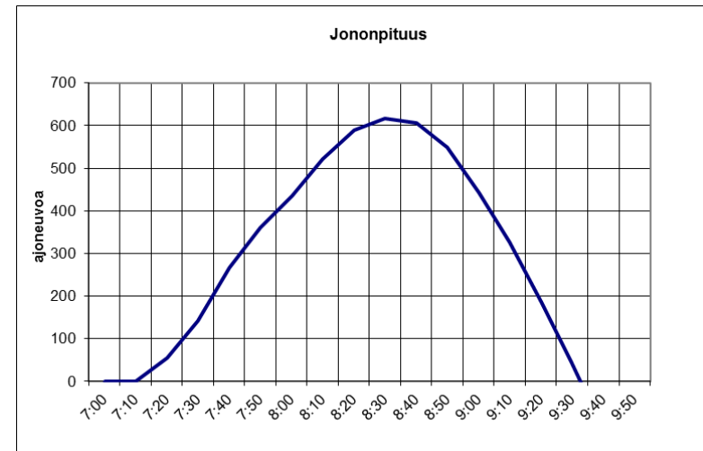
Esimerkki jonon muodostumisesta (Lahdenväylä, ve 3).
