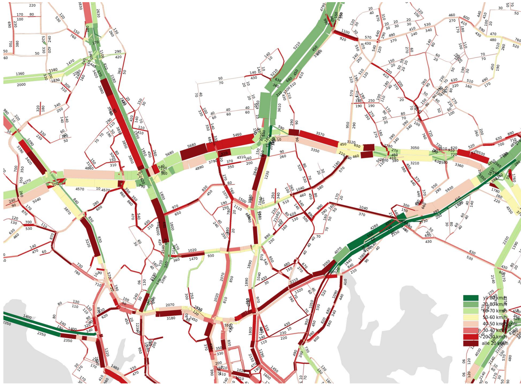
Autoliikenteen määrät ja sujuvus, AHT 2050 ve Tb (Tuusulanväyläbulevardi).
