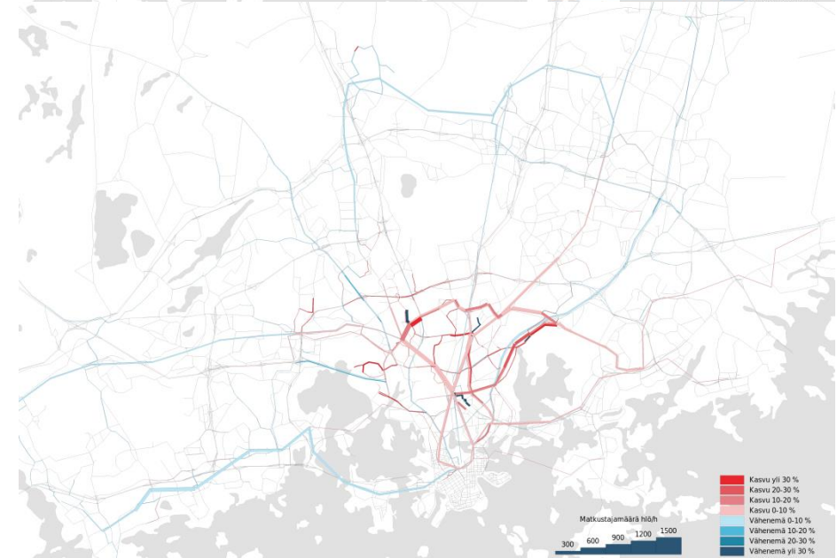
Vaikutukset tieliikenteen ja joukkoliikenteen määriin aamuruuhkassa, ve 2a.
