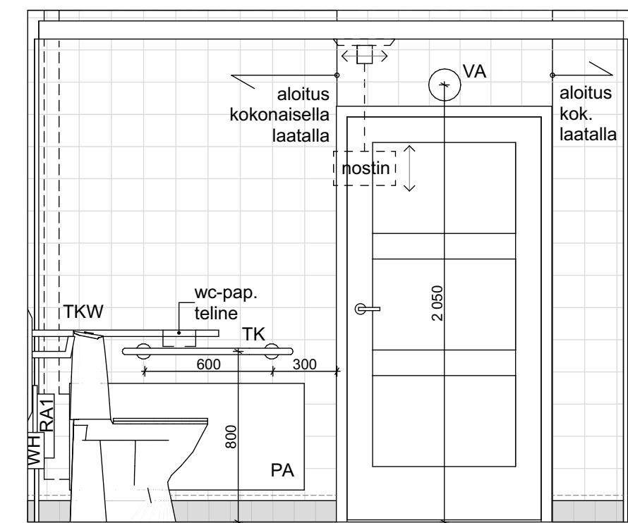
SEINÄPROJEKTIO F 221 LE-WC
