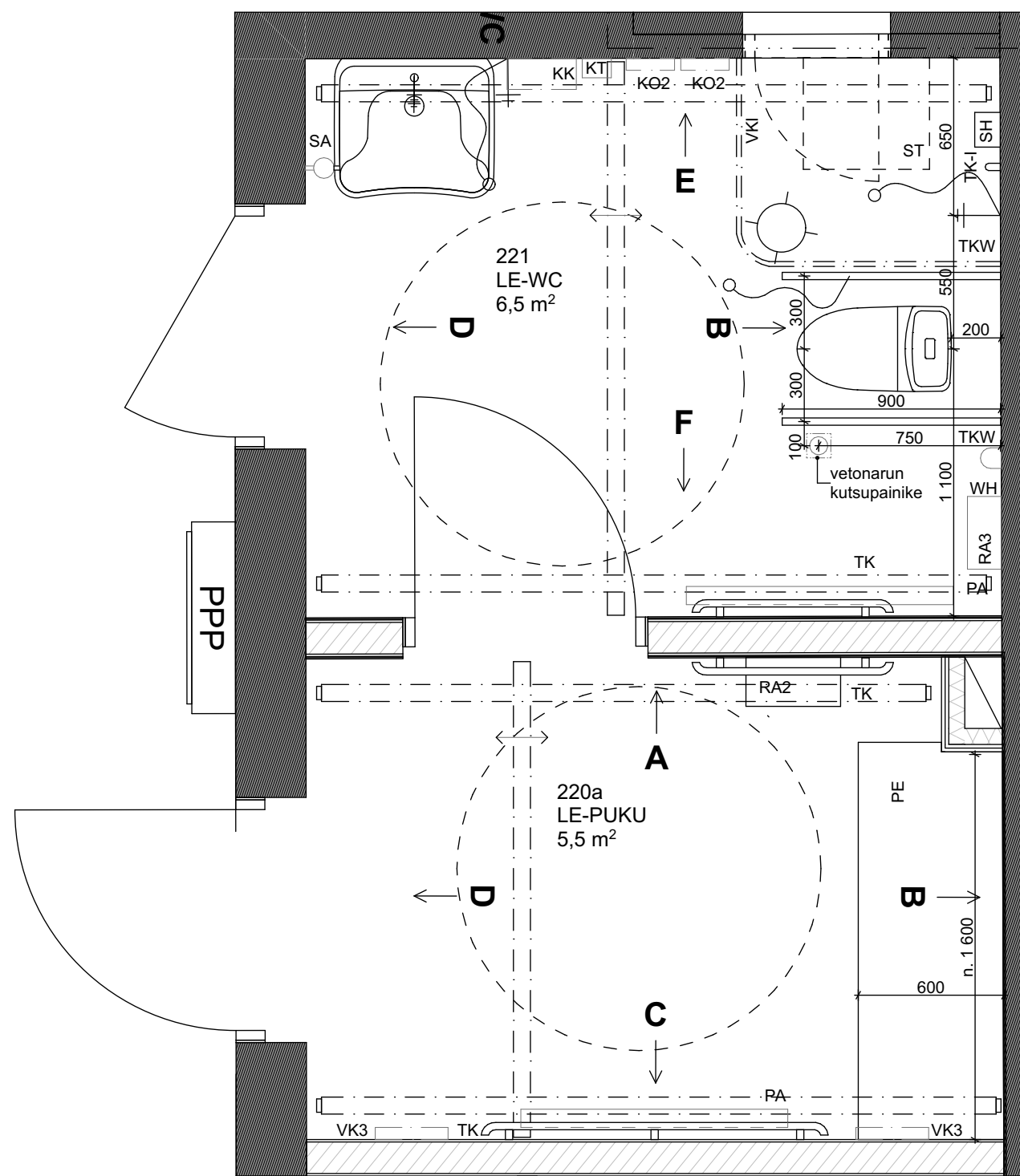
POHJAPIIRUSTUS 221 LE-WC JA 220a LE-PUKU
