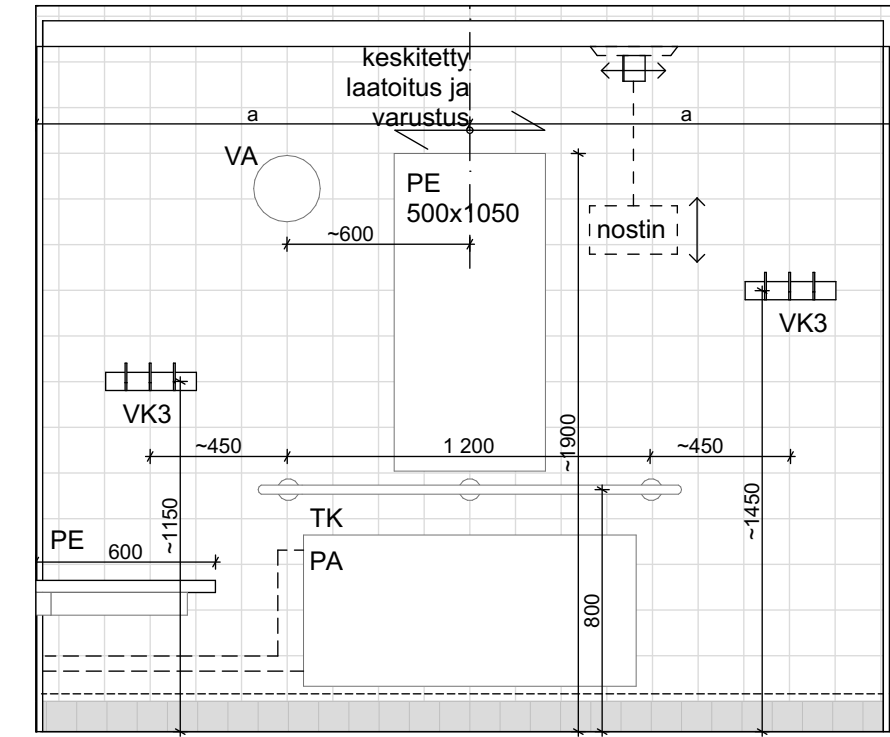
SEINÄPROJEKTIO C 220a LE-PUKU
