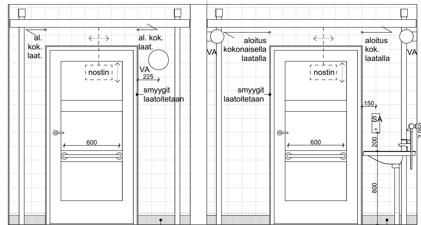
SEINÄPROJEKTIO D 220a LE-PUKU
