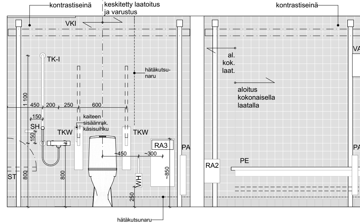
SEINÄPROJEKTIO B 221 LE-WC
