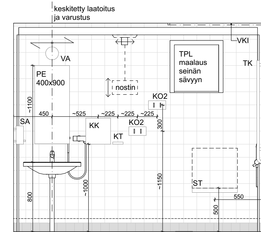
SEINÄPROJEKTIO E 221 LE-WC
