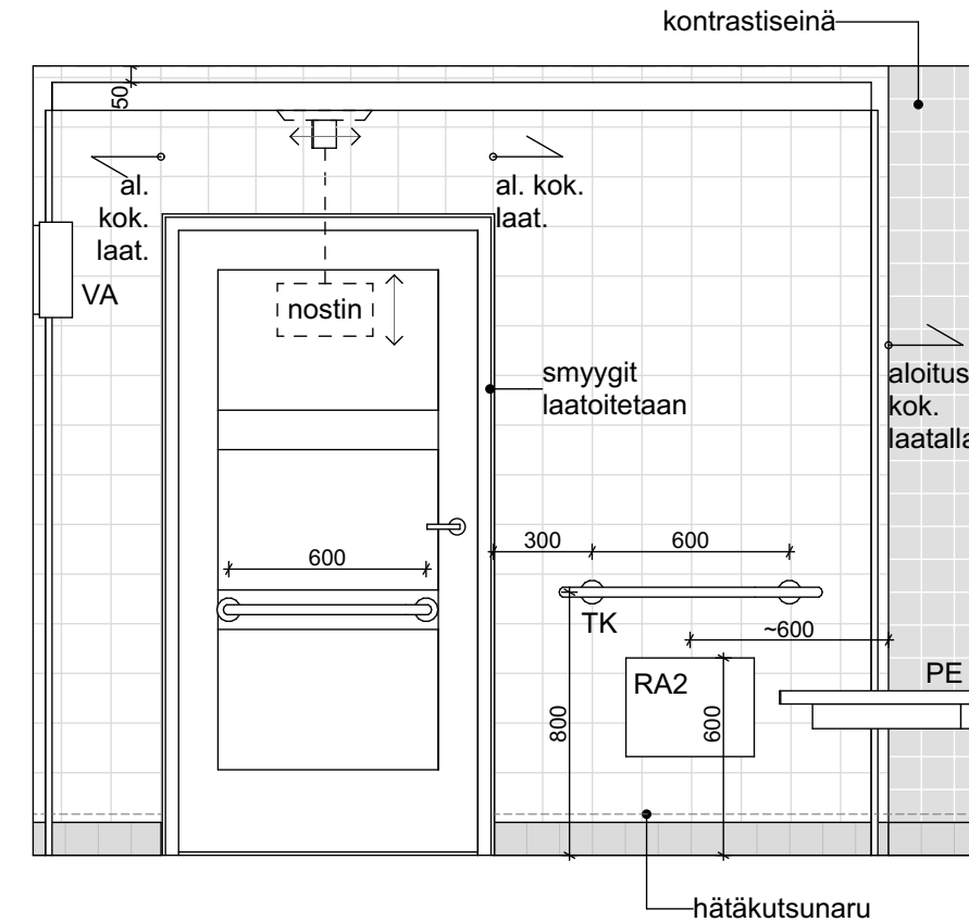
SEINÄPROJEKTIO A 220a LE-PUKU
