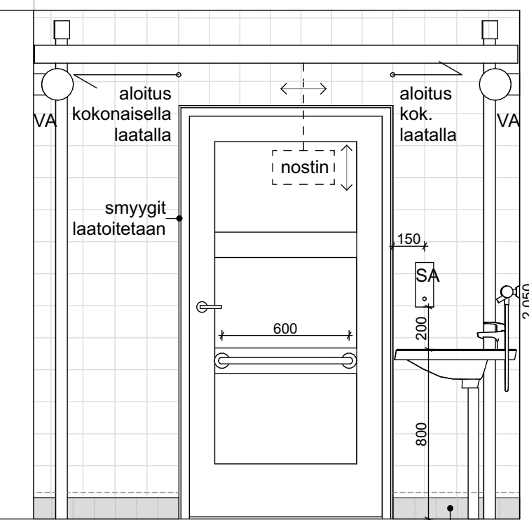
SEINÄPROJEKTIO D 221 LE-WC
