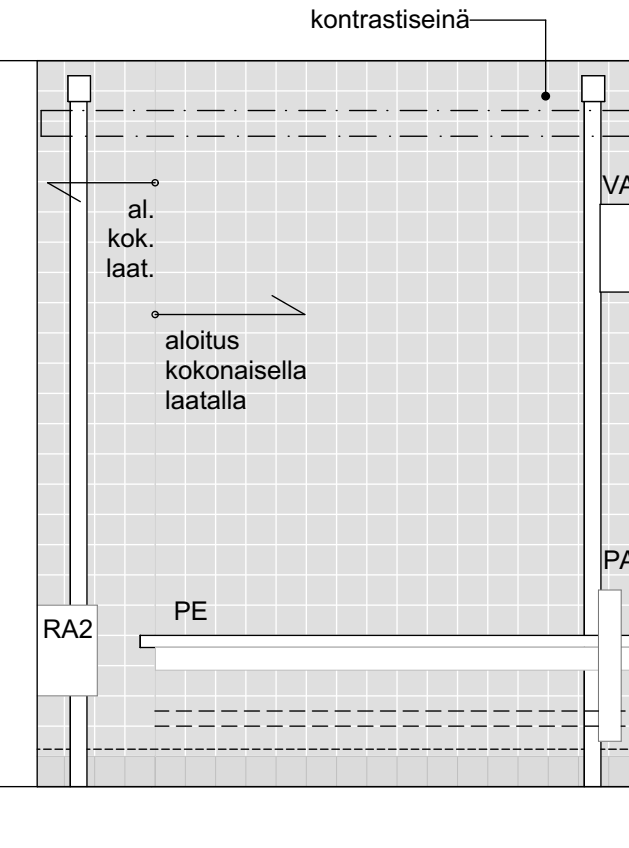
SEINÄPROJEKTIO B 220a LE-PUKU
