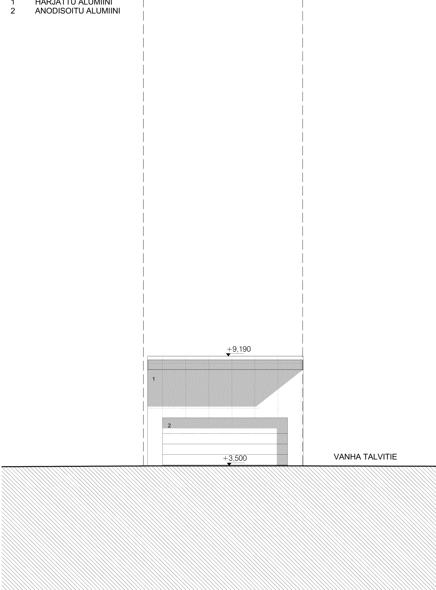
Ajoluiskan julkisivu Vanhalle Talvitielle 1:100
